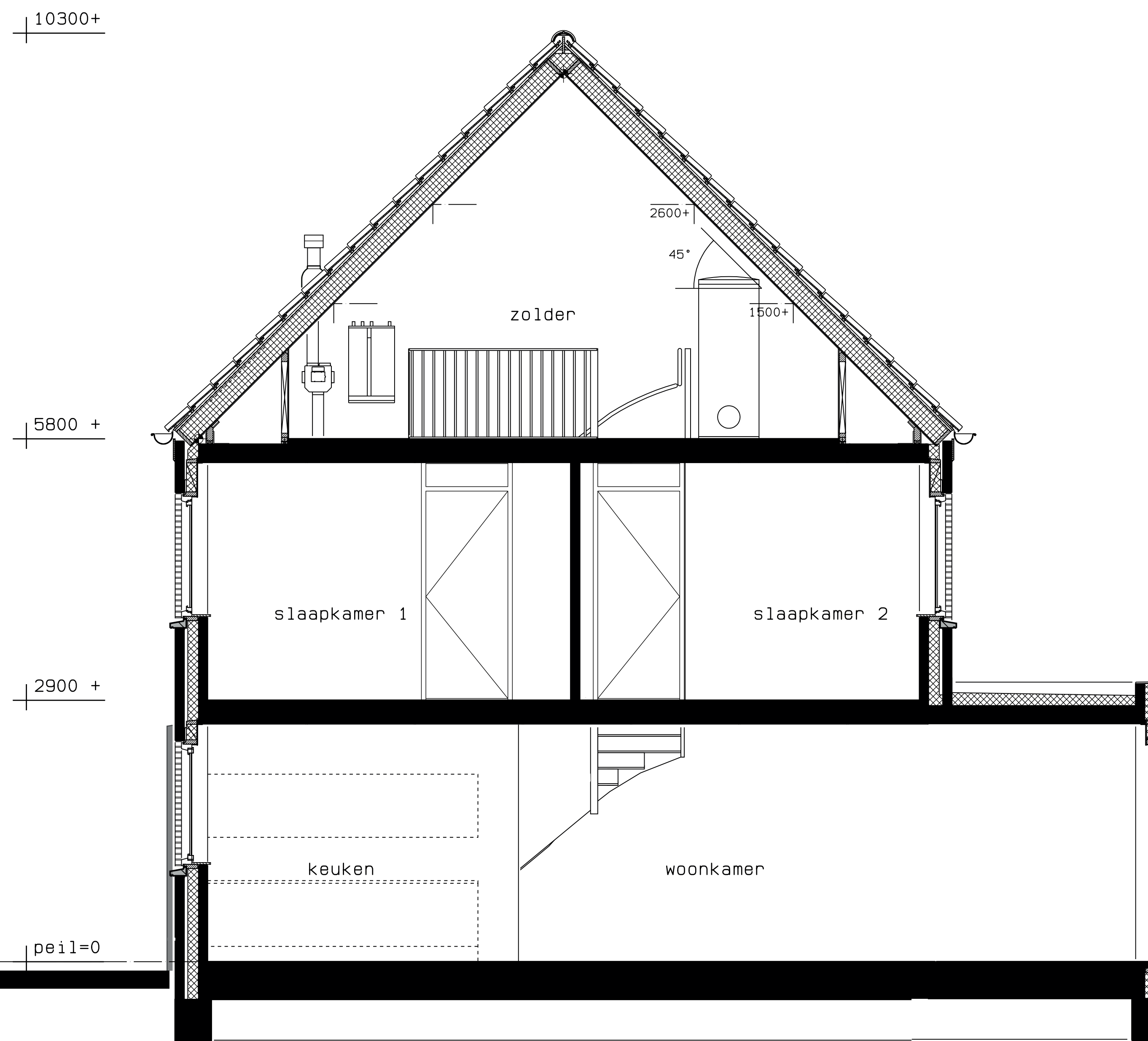
optie aanbouw 2,2m doorsnede
