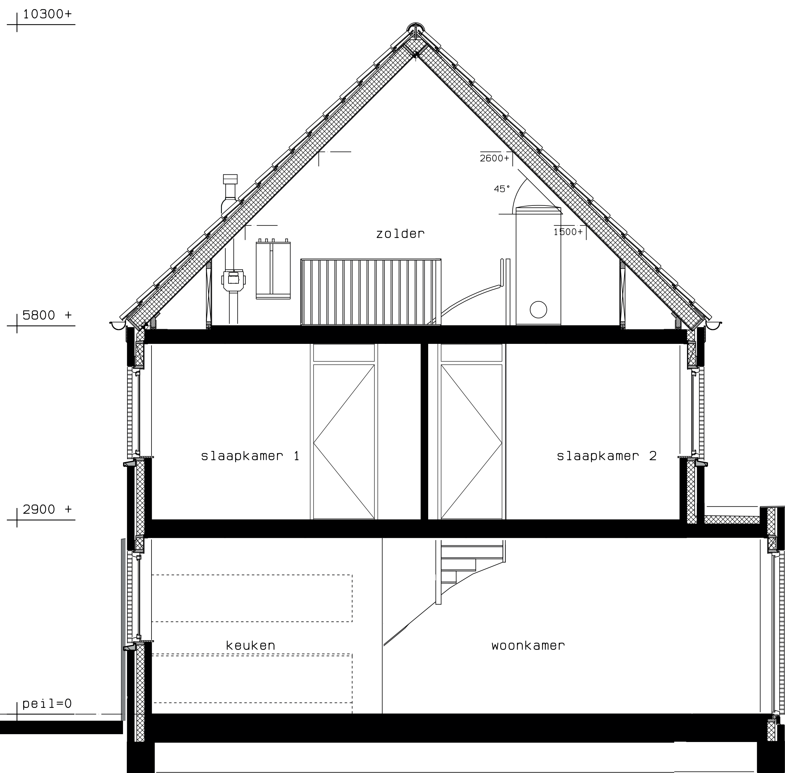
optie aanbouw 1,2m doorsnede
