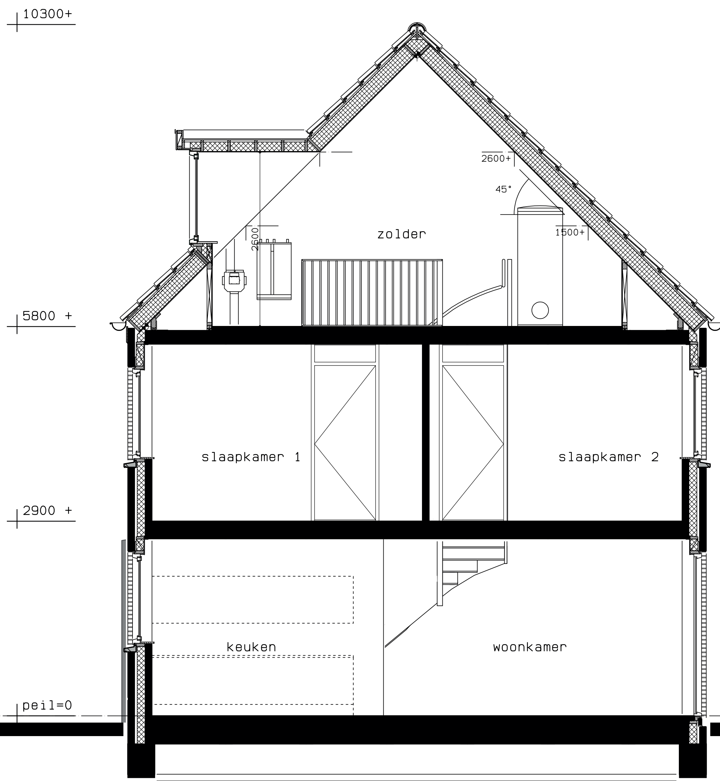
optie dakkapel voorgevel doorsnede
