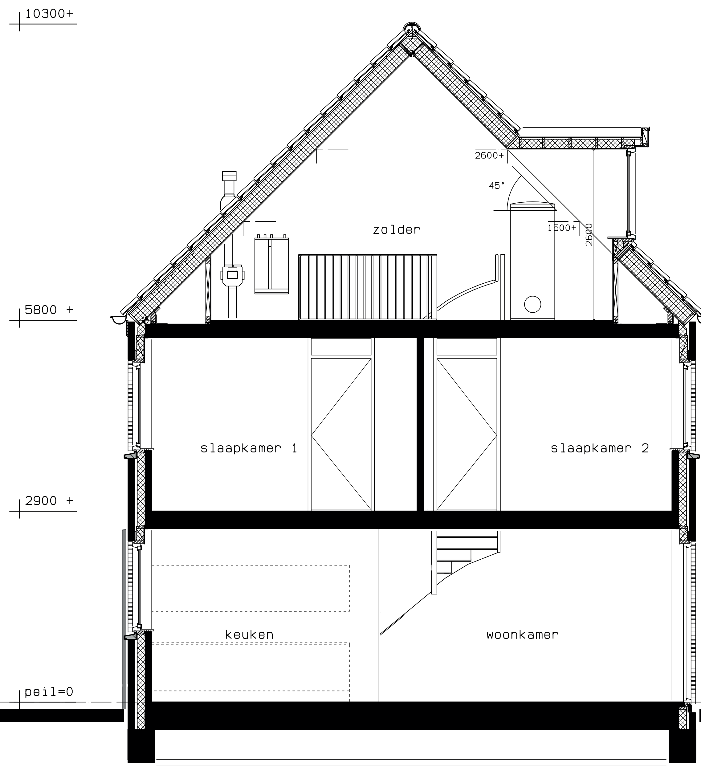
optie dakkapel achtergevel doorsnede
