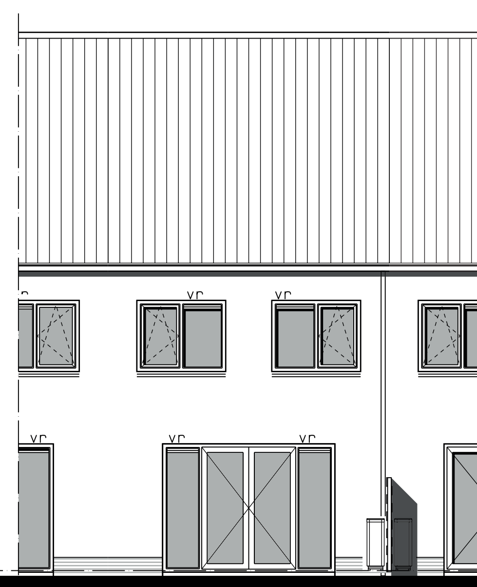
optie dubbele deuren achtergevel
