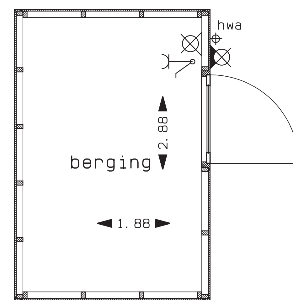
bouwnummer A7 plattegrond
